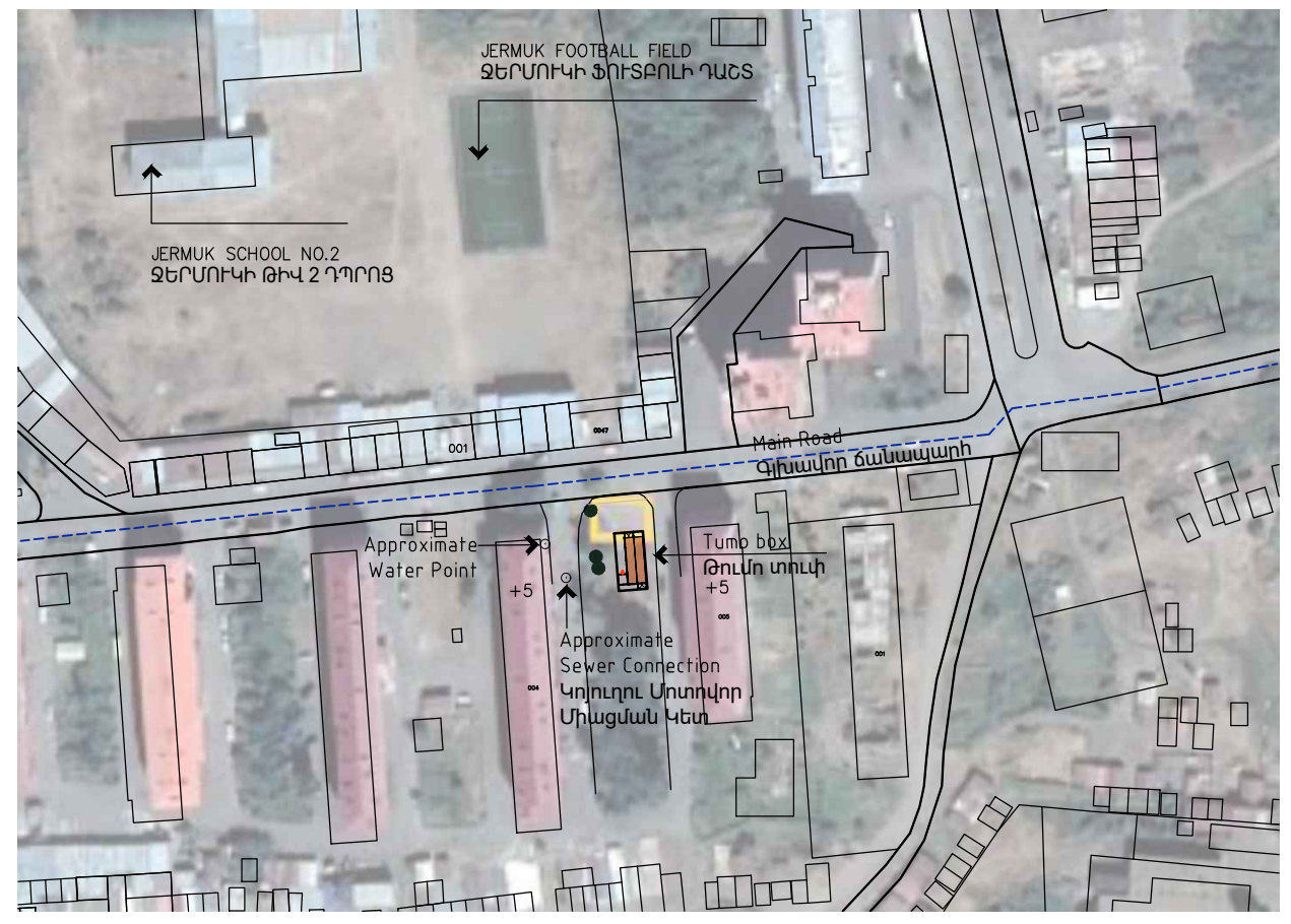
2 ԻՐԱԿԻՃԱԿԱՅԻՆ ՀԱՏԱԿԱԳԻԾ 2 SITUATION PLAN 1:2000@ A3
